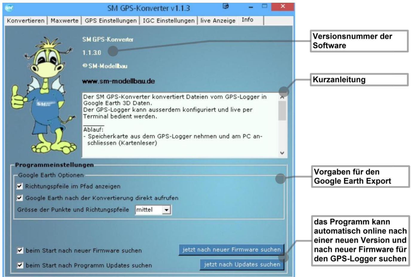
Abbildung 7: Reiter "Info"
