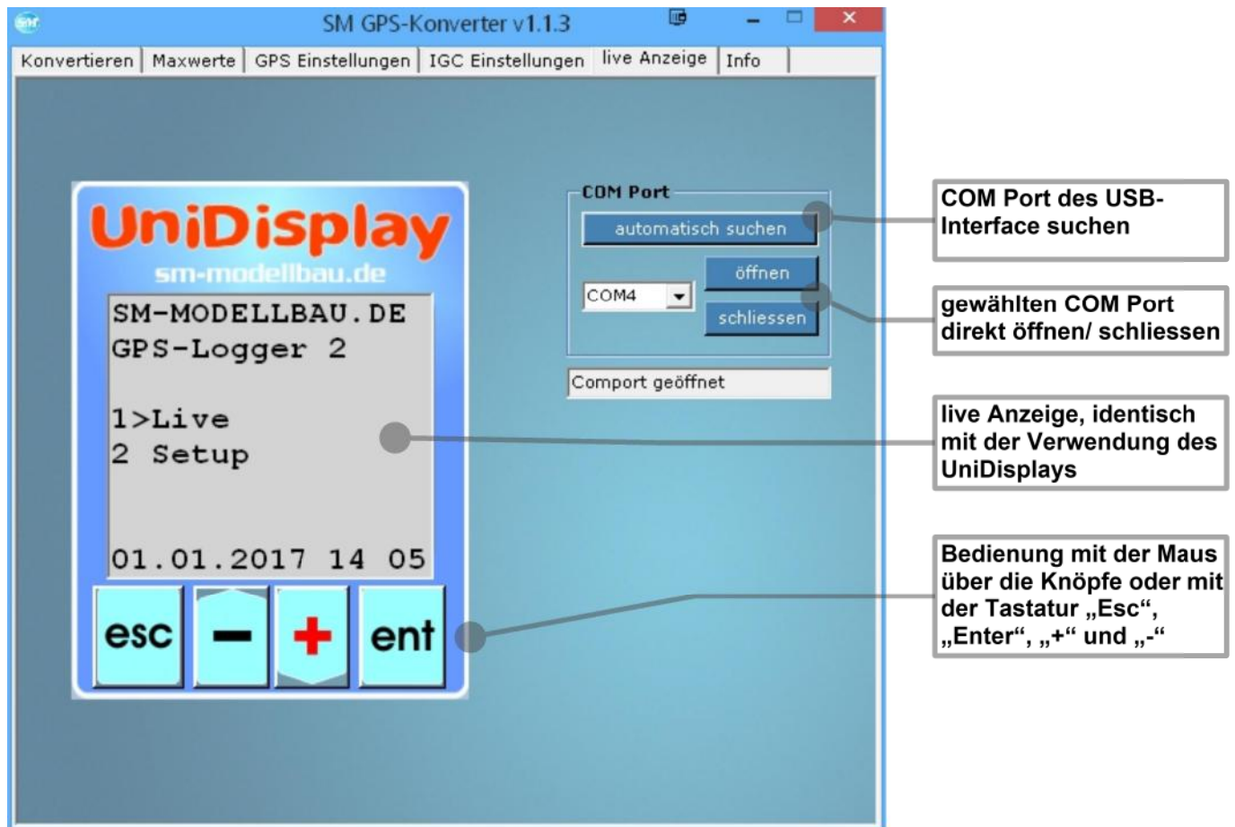
Abbildung 6: Reiter "Terminal"
